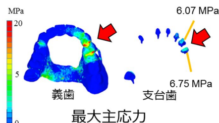
図4: 症例の有限要素解析結果
