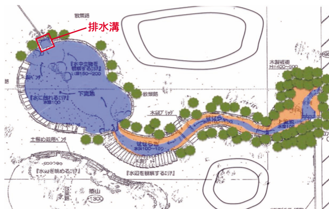
図20 改善案の具体例、水辺の埋立て（茶色部分）。右側「上流池」の小規模化、「せせらぎ」の川幅減少、水域近傍への植樹を示す。
