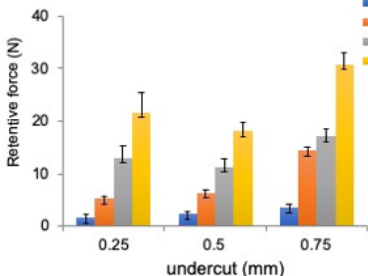
図 20 エステショットの初期維持力
