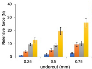
図 17 バルブラストの初期維持力
