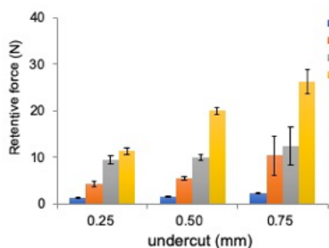
図 18 アミド・デ・ショットの初期維持力
