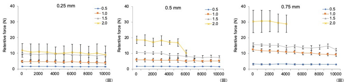
図 23 エステショットブライトにおけるの維持力の経過 (左からアンダーカット量 0.25, 0.5, 0.75 mm)
