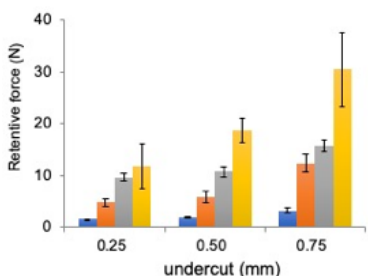
図 19 エステショットブライツの初期維持力
